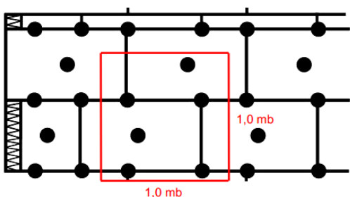
Schemat układu kołków w strefie przynaróżnikowej -6 sztuk /m2 (budynek do 5-kondygnacji)
