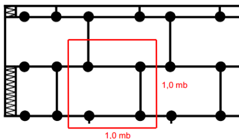
Schemat układu kołków w strefie przynaróżnikowej -6 sztuk /m2 (budynek do 5-kondygnacji)
