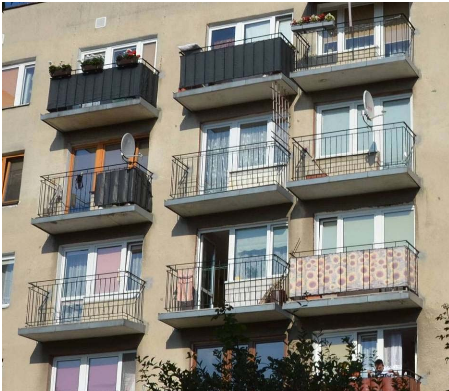
FOT.2. Widok na balkony. Płyta balkonu oraz balustrady w dość dobrym stanie technicznym.
